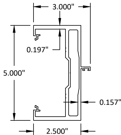
15 DOOR MULLION O/P
